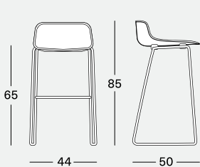
P 8360, U 8361 Sgabello basso slitta Bar stool low sled base Tabouret bas base sur luge Hocker, niedrig
