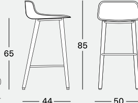
P 8340, U 8341 Sgabello basso quattro gambe legno Bar stool low four wooden legs Tabouret bas jambes en bois Hocker, niedrig, mit Holzbeinen
