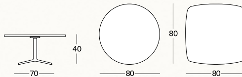
P011 Tavolo basso, Piano MDF h. 40 cm Side-table, Top in MDF h. 40 cm Table d'appoint, Plateau MDF h. 40 cm Beistell-Tisch, MDF Platte h. 40 cm
