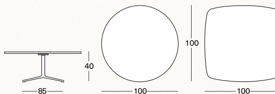
P031 Tavolo basso, Piano MDF h.40, Piano impiallacciato h. 40 cm Side-table, Top in MDF h. 40 cm, Veneered top h. 40 cm Table d'appoint, Plateau MDF h. 40 cm, Plateau contre-plaqué h. 40 cm Beistell-Tisch, MDF Platte h. 40 cm, Platte, furniert h. 40 cm
