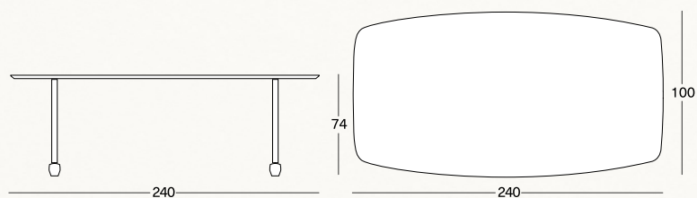
P060 Tavolo, Piano MDF h.74, Piano impiallacciato h. 74 cm Table, Top in MDF h. 74 cm, Veneered top h. 74 cm Table, Plateau MDF h. 74 cm, Plateau contre-plaqué h. 74 cm Tisch, MDF Platte h. 74 cm, Platte, furniert h. 74 cm
