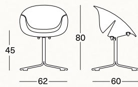
Ⓟ 4020, Ⓛ 4021 Base centrale fissa Central base Base centrale fixe 4-strahliges Fusskreuz, nicht drehbar
