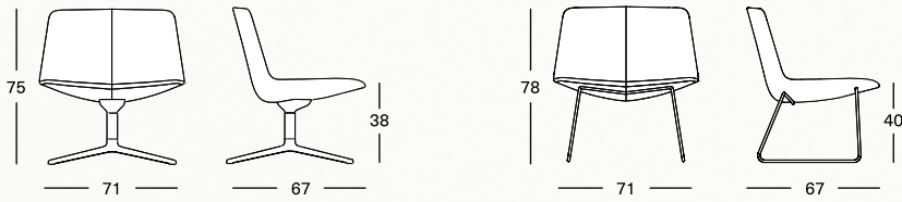
Ⓢ SL01 Base girevole Swivel base Base pivotante 4-strahliges Fusskreuz, drehbar
