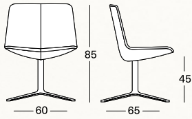
① SM01 Base girevole Swivel base Base pivotante 4-strahliges Fusskreuz, drehbar
