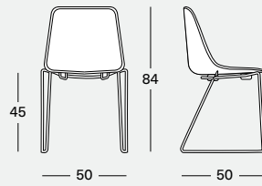
P 6050, U 6051 Base a slitta Sled base Base sur luge Kufengestell
