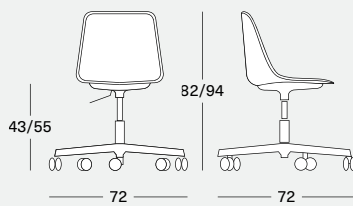
P 6530, U 6531 Cinque razze con ruote, girevole, con meccanismo a gas Swivel aluminium base with castors and gas lift mechanism Base pivotante sur roulettes 5-strahliges Fusskreuz auf Raedern, drehbar, mit Liftgasmechanismus
