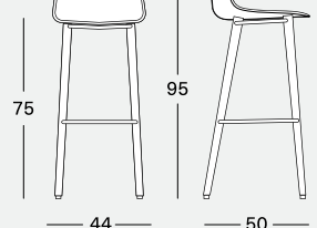
P 8350, U 8351 Sgabello alto quattro gambe legno Bar stool high four wooden legs Tabouret haut avec jambes en bois Hocker, hoch, mit Holzbeinen
