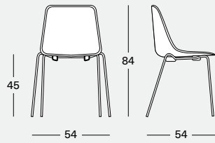
P 6010, U 6011 Quattro gambe metallo Four metal legs Quatre jambes Vier Beine
