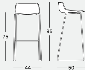
P 8370, U 8371 Sgabello alto slitta Bar stool high sled base Tabouret haut base sur luge Hocker, hoch
