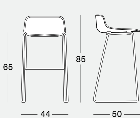
P 8360, U 8361 Sgabello basso slitta Bar stool low sled base Tabouret bas base sur luge Hocker, niedrig
