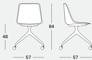
P 6640, U 6641 Trespolo con ruote, fisso Trestle base fix with castors Base non pivotante sur chevalet avec roulettes Fusskreuz fest, auf Raedern
