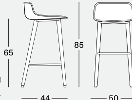
P 8340, U 8341 Sgabello basso quattro gambe legno Bar stool low four wooden legs Tabouret bas jambes en bois Hocker, niedrig, mit Holzbeinen
