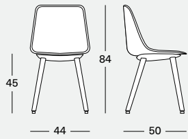
P 6040, U 6041 Quattro gambe legno Four wooden legs Quatre jambes bois Vier Holzbeine
